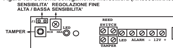
Figura 1B: Schema collegamento morsettiera (RK600SMXX00A)
